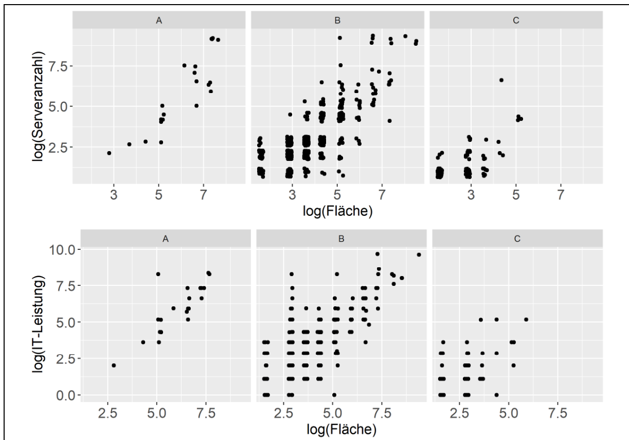
Abbildung 37: \log(\text{Serveranzahl}) und \log(\text{IT-Leistung}) in kW als Funktion der Nutzfläche für die Segmente A, B und C.
