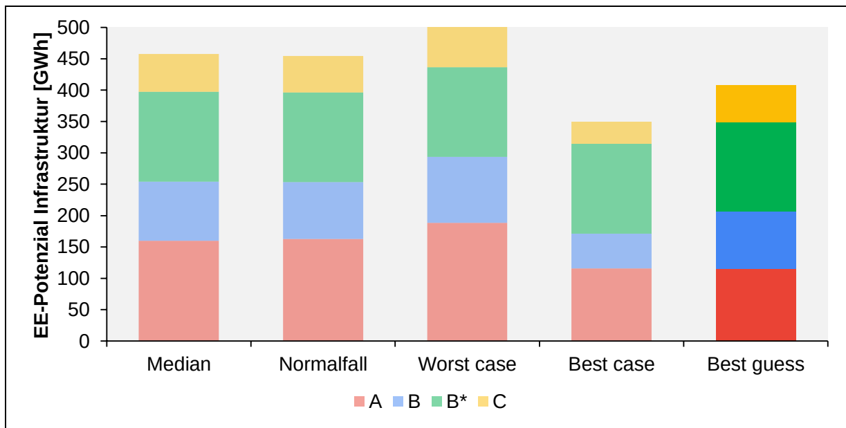
Abbildung 27: Infrastrukturseitige Energieeffizienzpotenziale anhand der verschiedenen Szenarien Median, Normalfall, Worst case, Best case sowie Best guess.
