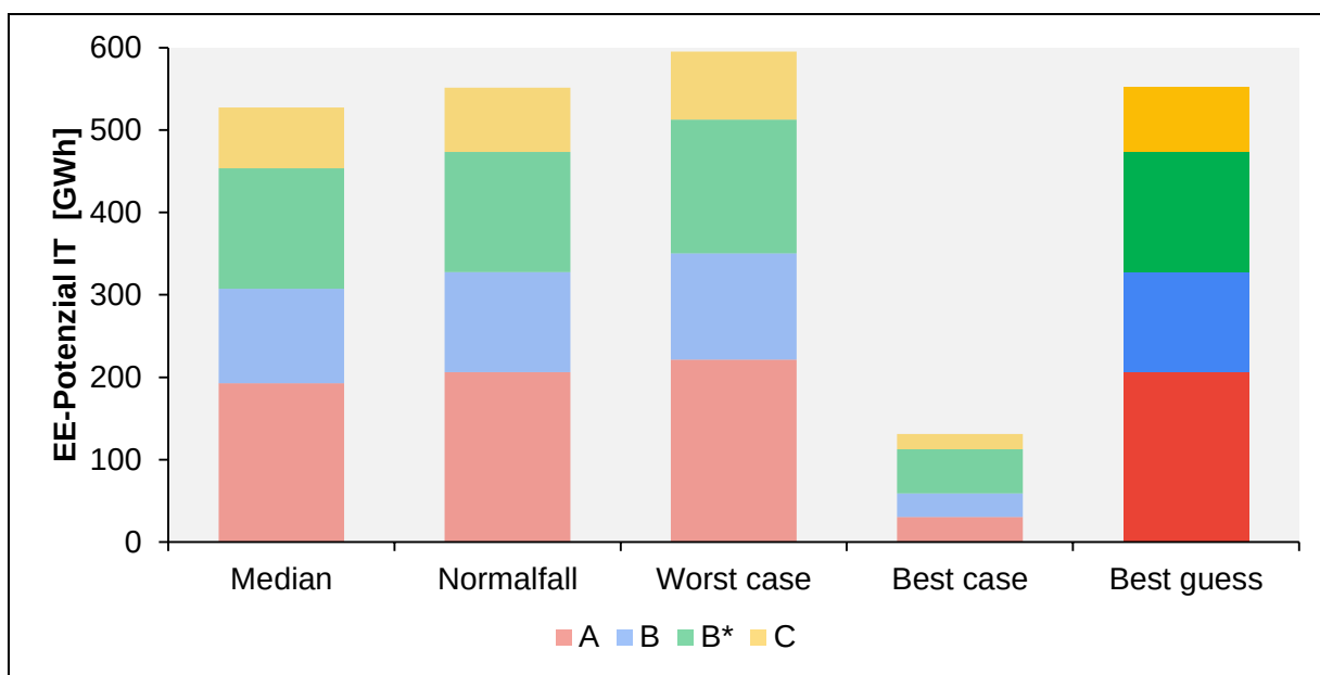
Abbildung 28: IT-seitige Energieeffizienzpotenziale anhand der verschiedenen Szenarien Median, Normalfall, Worst case, Best case sowie Best guess.
